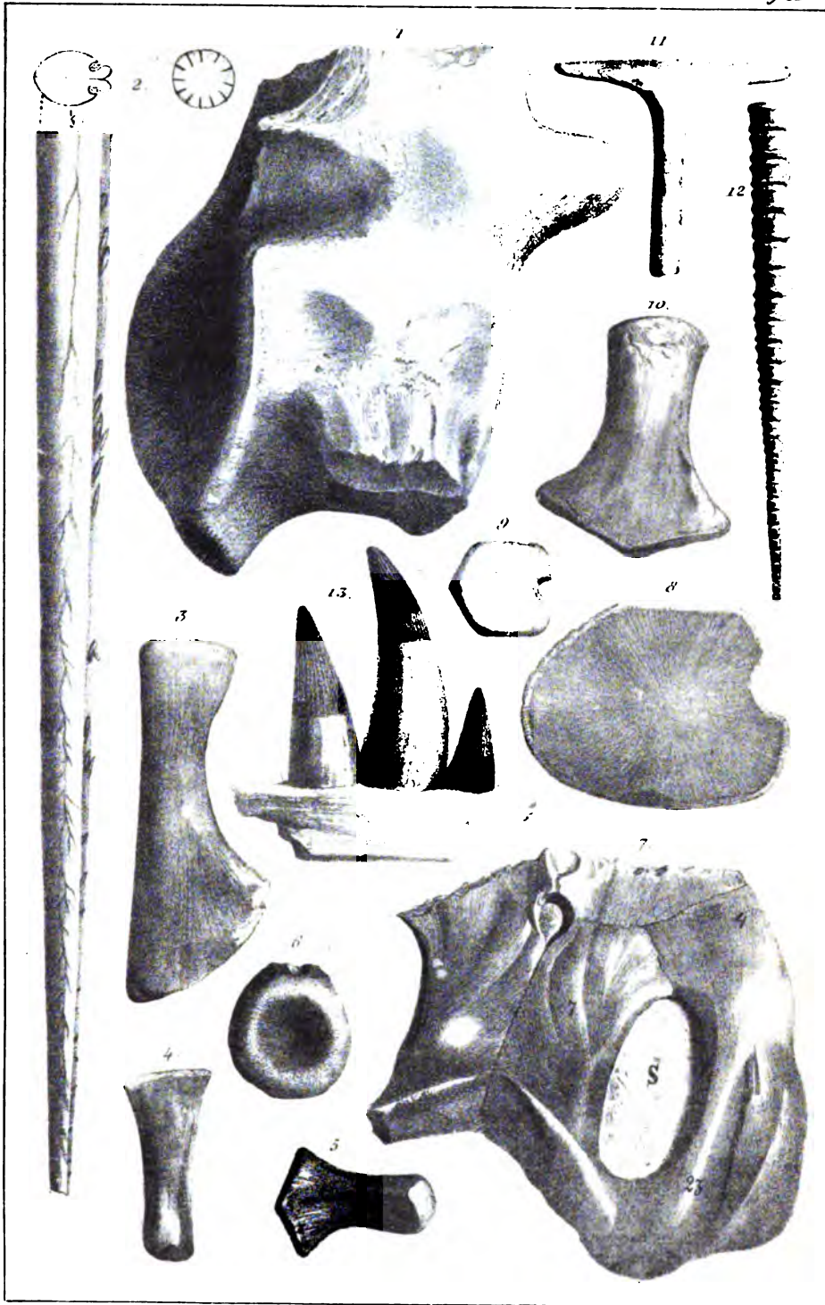
Wiesbaden, Jura.
